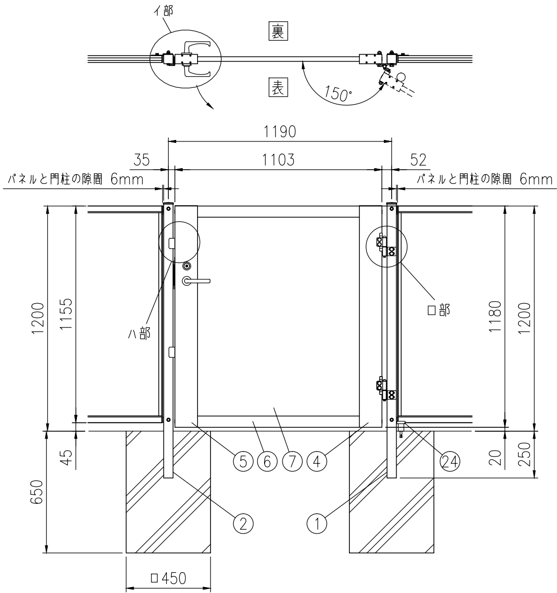
組立図 (1/20) 吊元右側、表開きの時 注) 基礎の大きさは参考寸法です。
