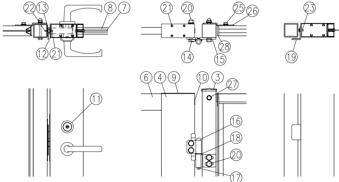
イ部詳細図 (1/8) ロ部詳細図 (1/8) ハ部詳細図 (1/8)
