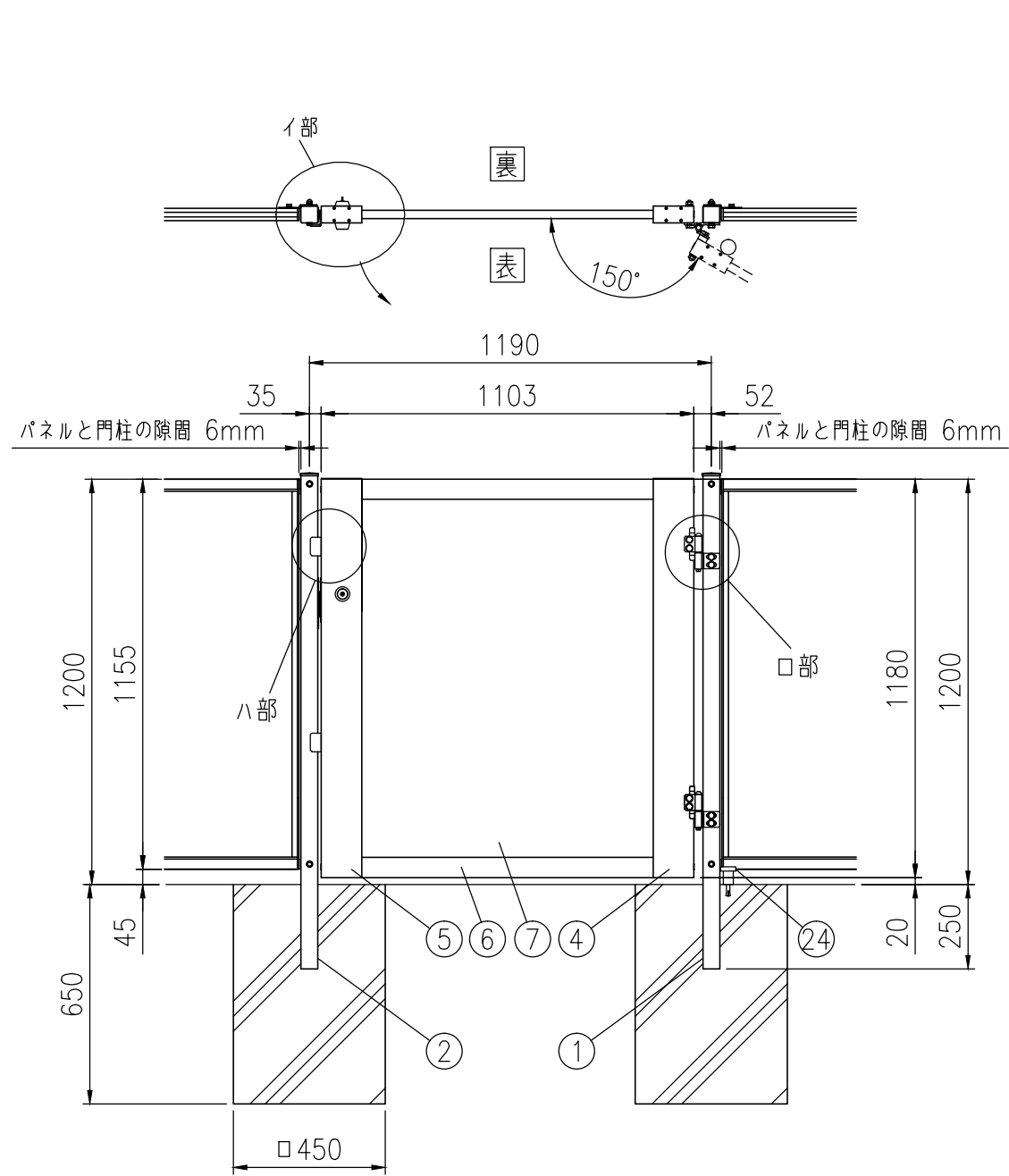
組立図 (1/20) 吊元右側、表開きの時 注) 基礎の大きさは参考寸法です。
