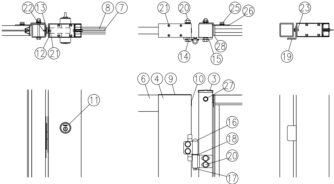
イ部詳細図（1/8）
