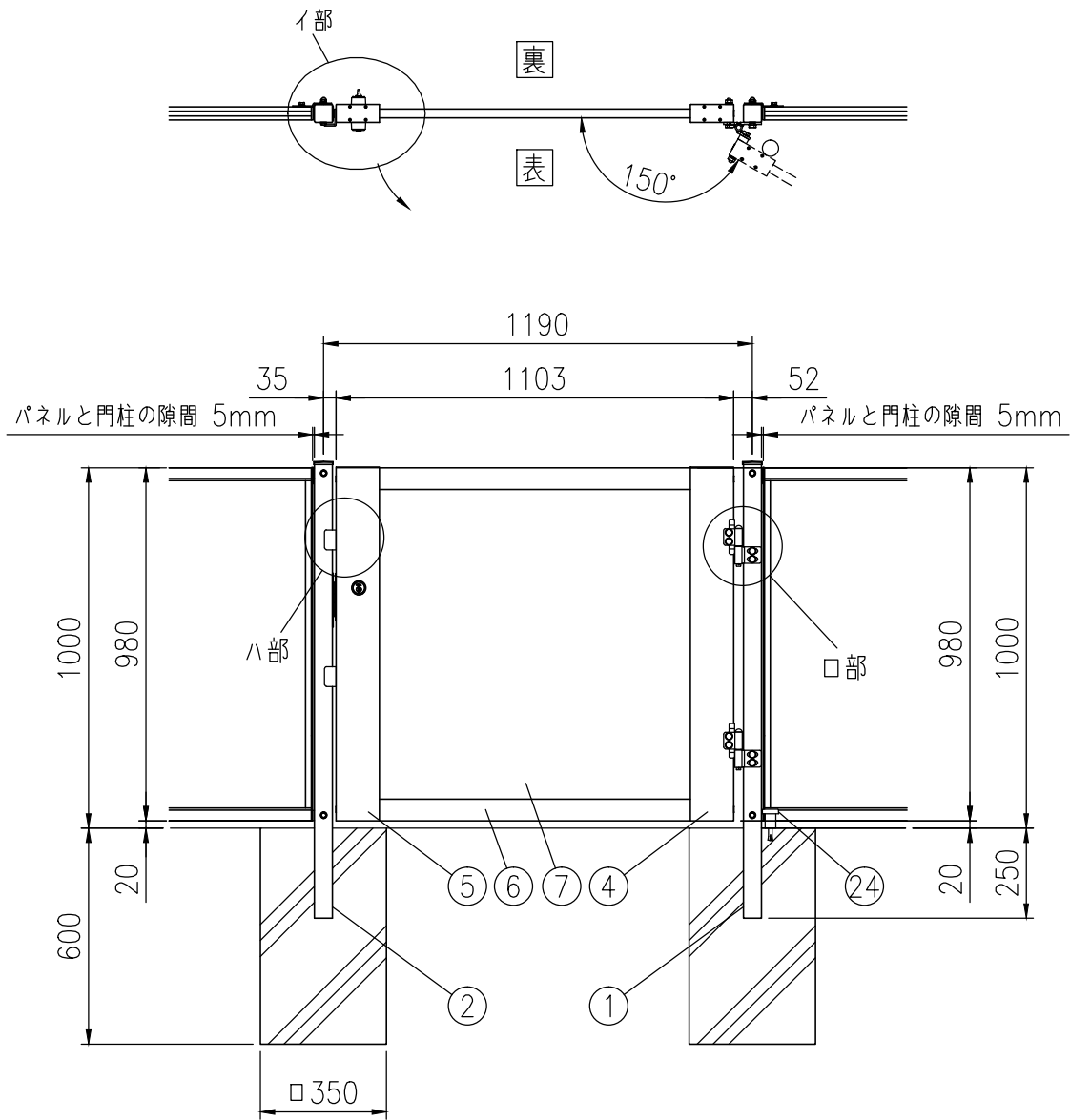
組立図（1/20）
