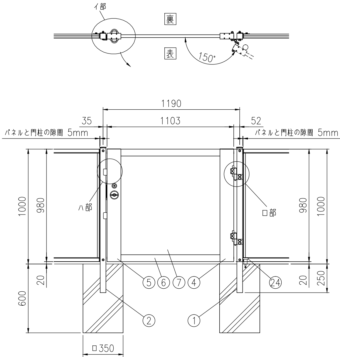
組立図（1/20）
