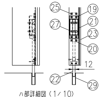
H部分詳細図 (1/10)
