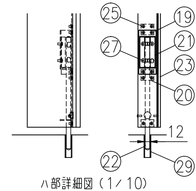
ハ部詳細図 (1/10)
