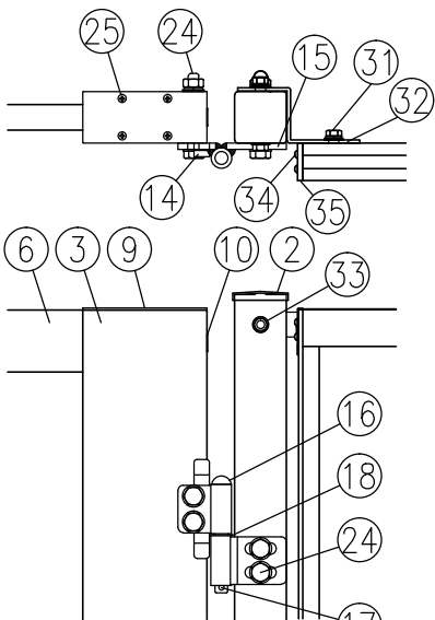
ロ部詳細図 (1/8)
