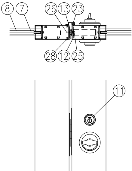
イ部詳細図 (1/8)
