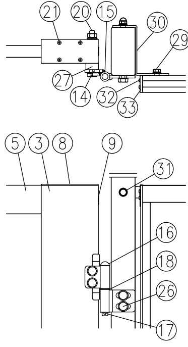
□部詳細図 (1/8)
