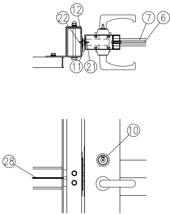
イ部詳細図 (1/8)
