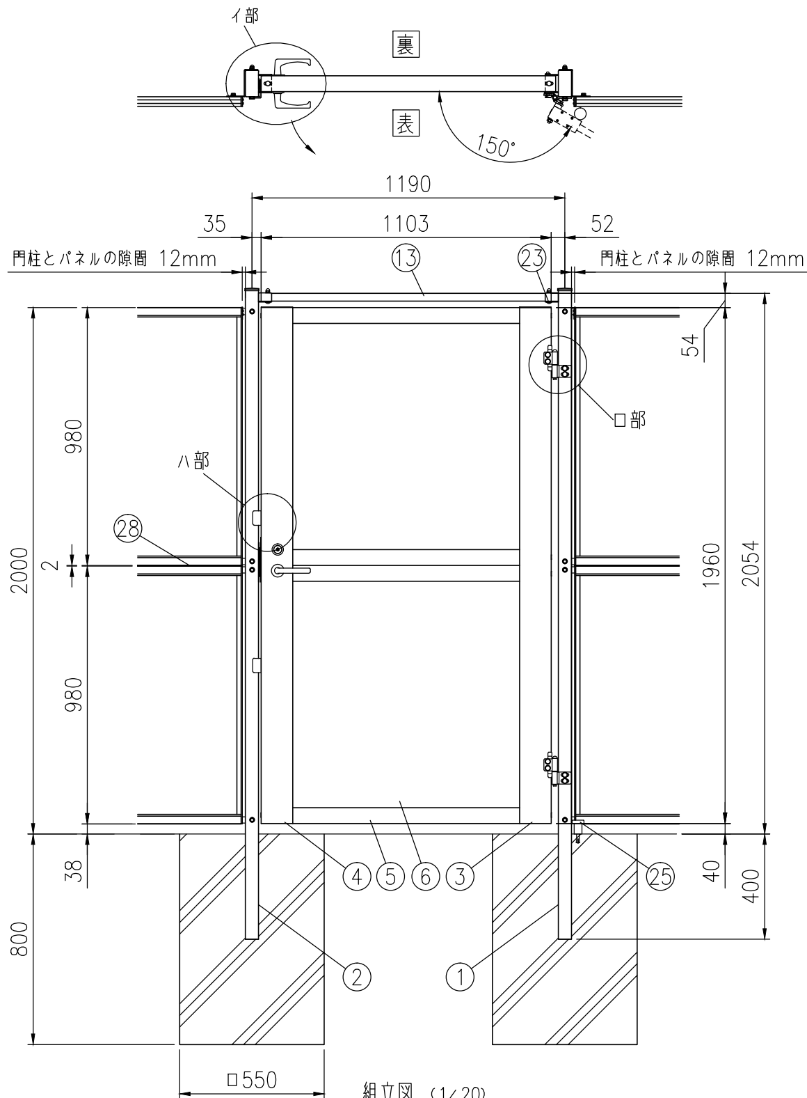
組立図 (1/20)
