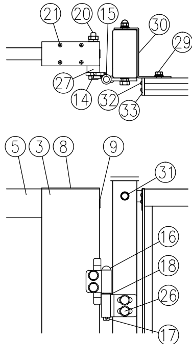
□部詳細図 (1/8)
