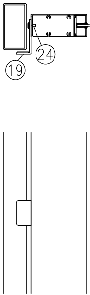
ハ部詳細図 (1/8)
