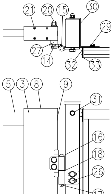
ロ部詳細図 (1/8)
