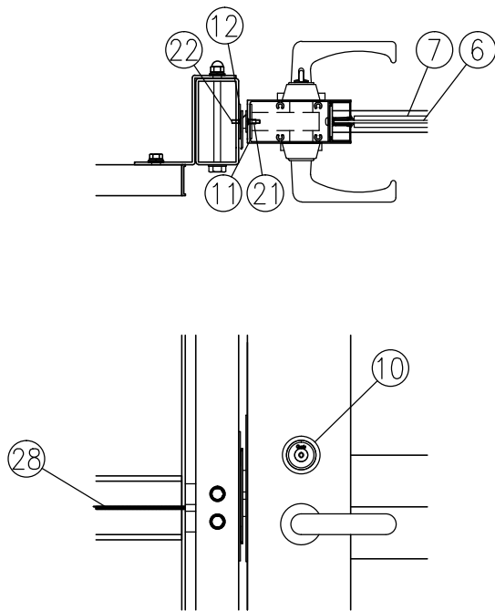
イ部詳細図 (1/8)
