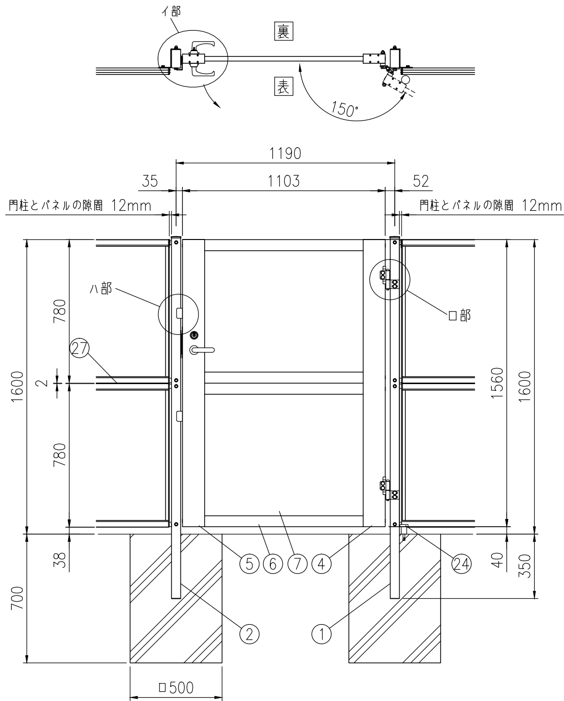
組立図 (1/20)
