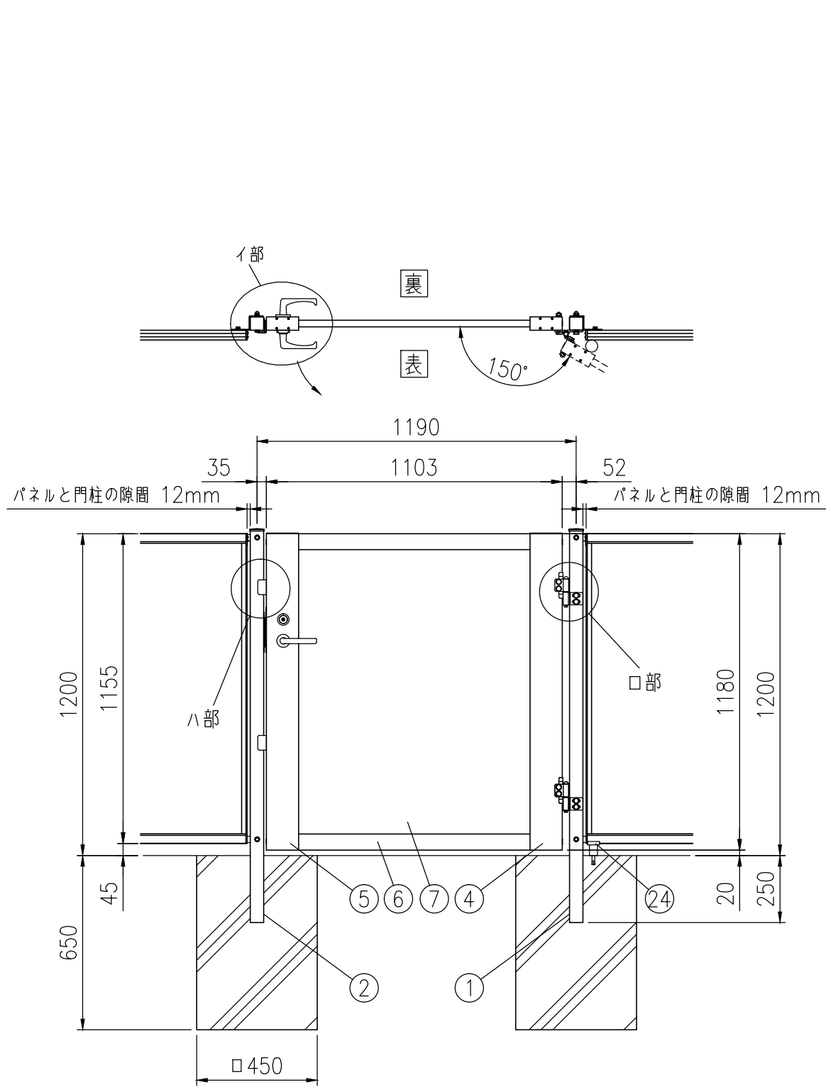
組立図 (1/20)
