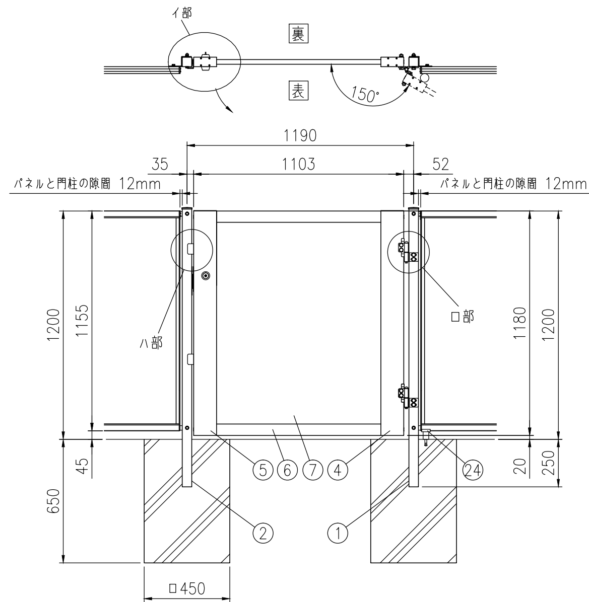
組立図 (1/20)
