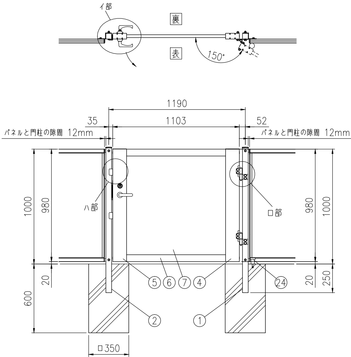
組立図（1/20）
