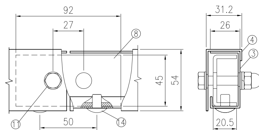
接続部部詳細図 (1/2)
