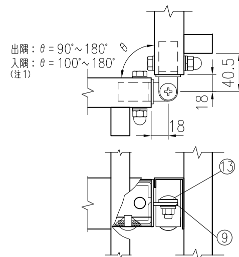
コーナー部施工例 (1/4)
