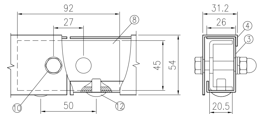
接続部部詳細図 (1/2)
