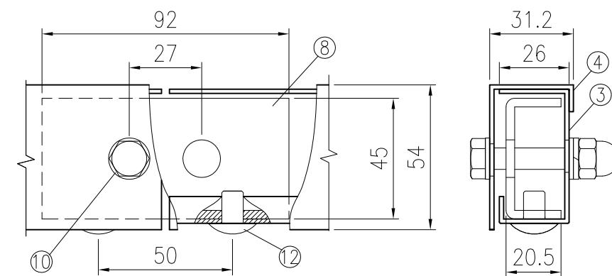
接続部部詳細図 (1/2)
