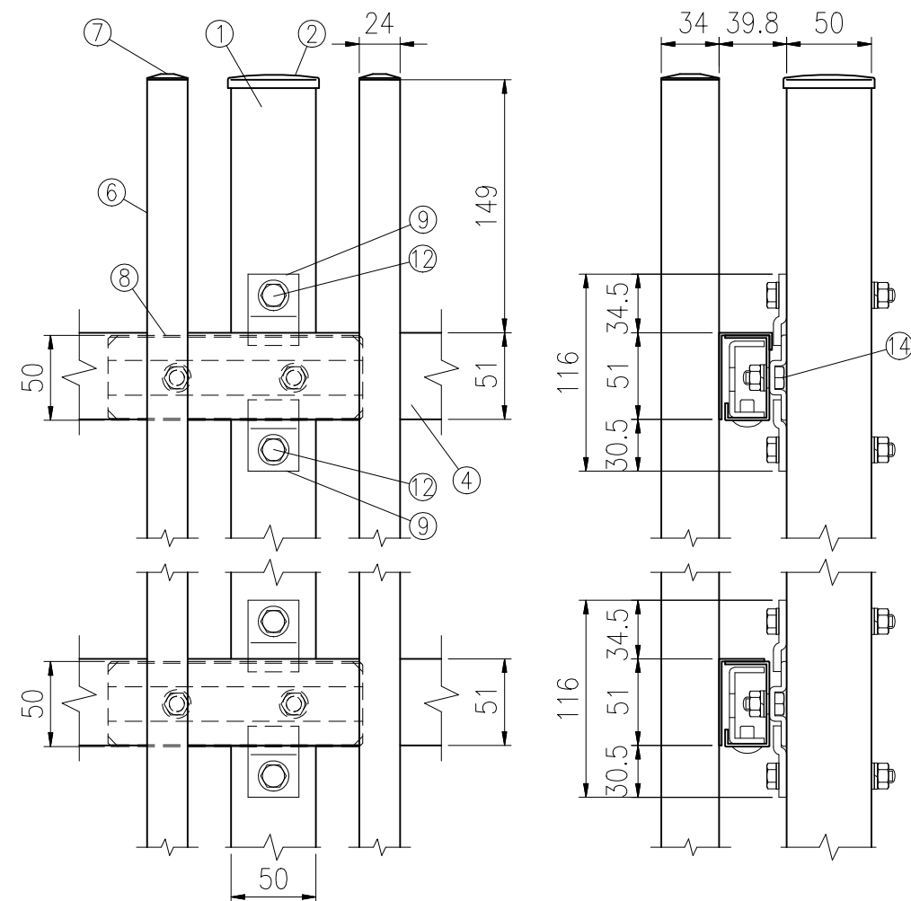
取付部詳細図 (1/4)
