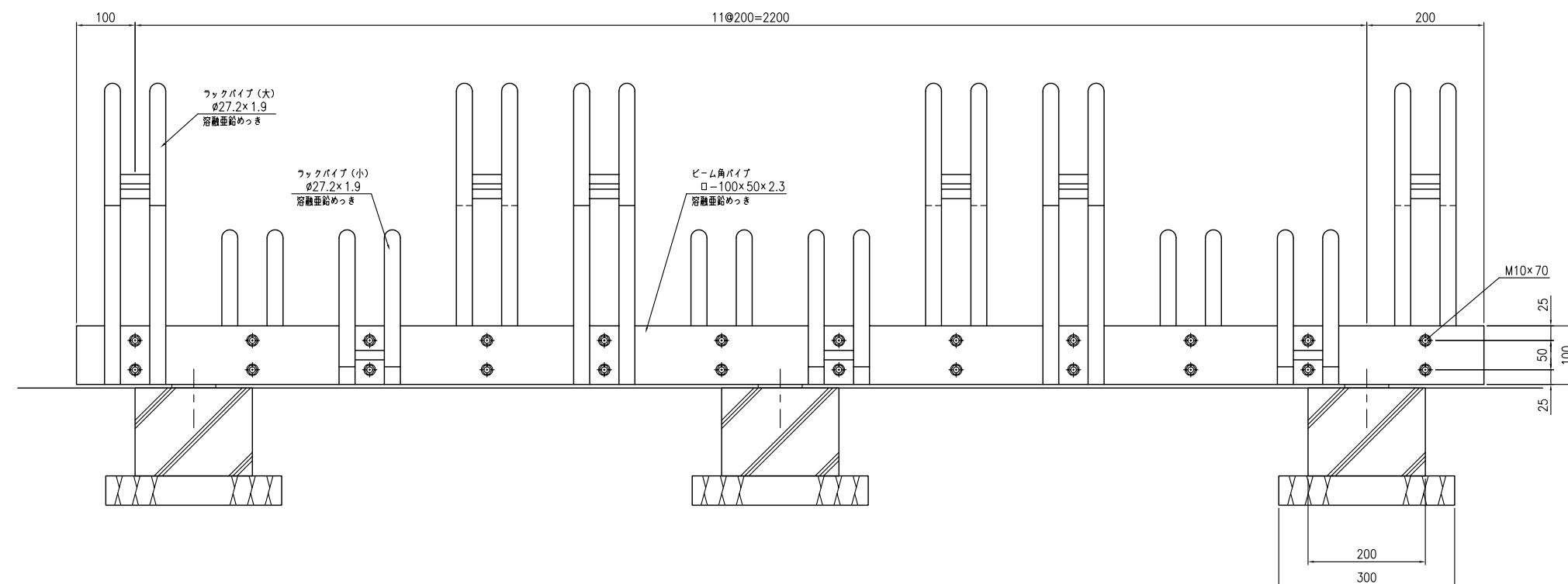
正面図 (S = 1 : 5)
