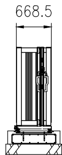
A-A矢視図
