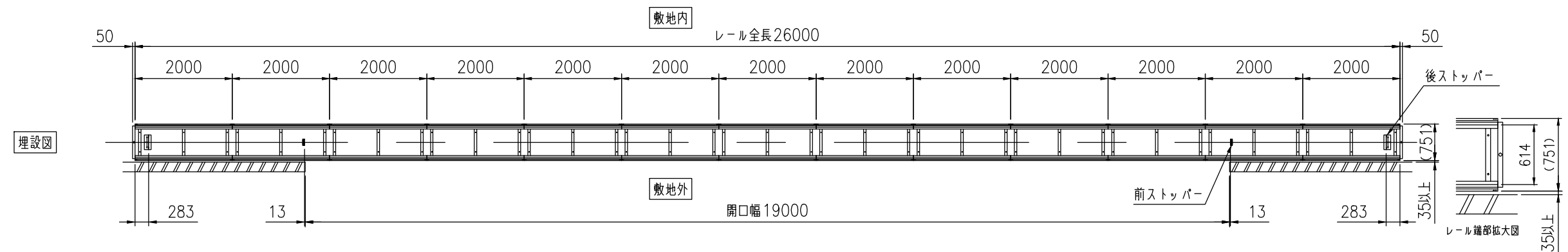
A-A矢视图
