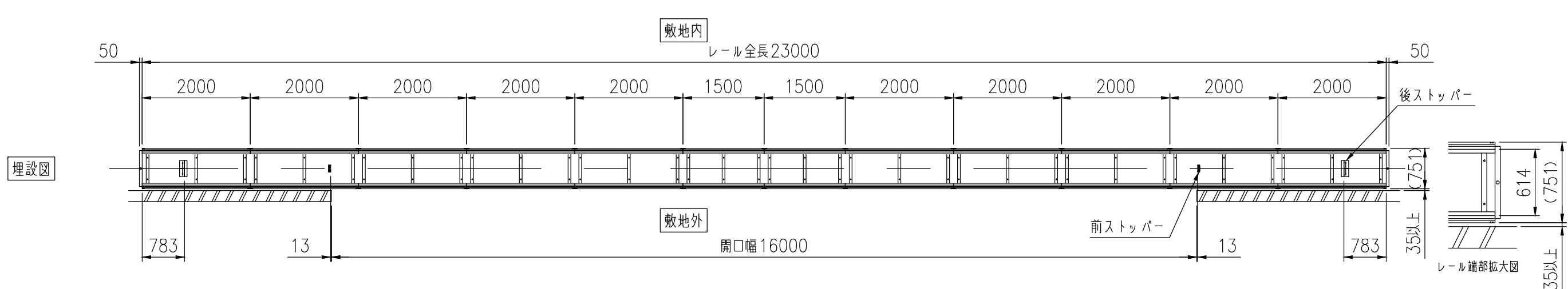
A-A矢视图
