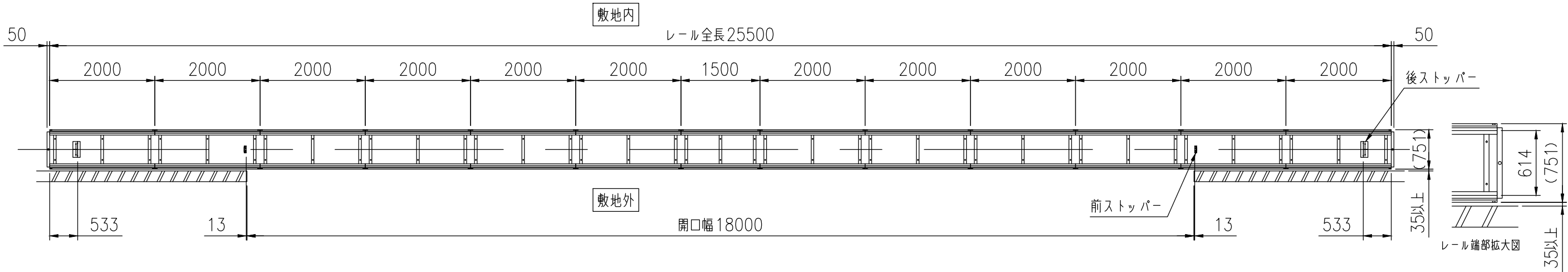
埋設図
