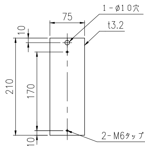
タソシバン詳細図 S = 1 / 5
