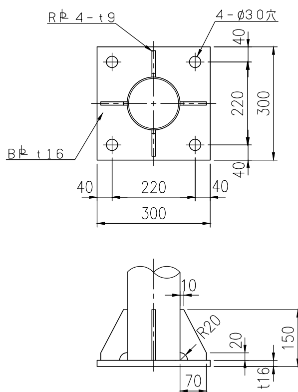
ベース部詳細図 S = 1 / 10
