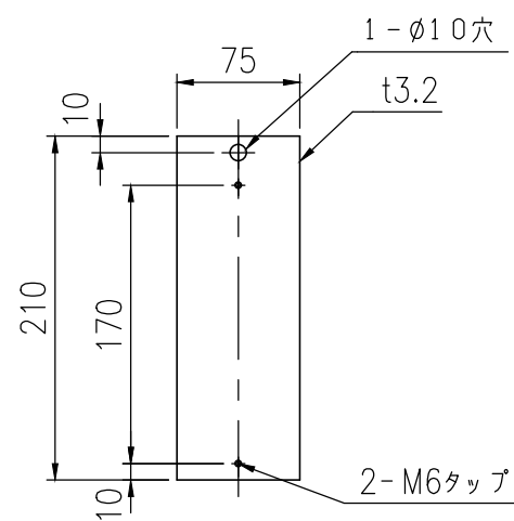
ベース部詳細図 S = 1 / 10
