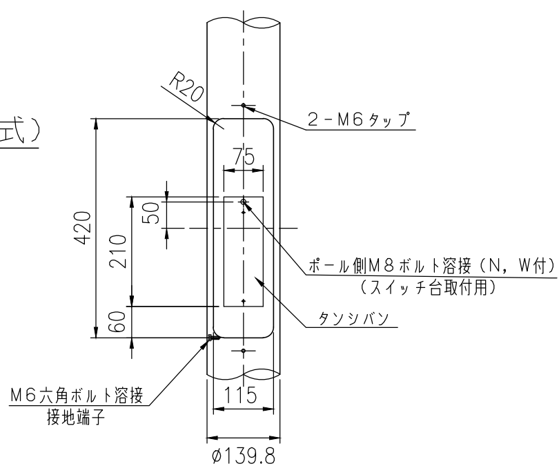
タソシバン詳細図 S = 1 / 5
