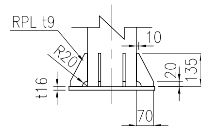
アソカーボルト詳細図 S=1/15
