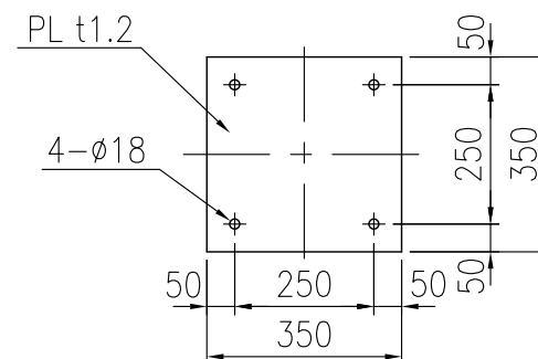
アソカーゲージ詳細図 S=1/15
