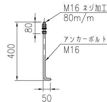
アソカーゲージ詳細図 S=1/15
