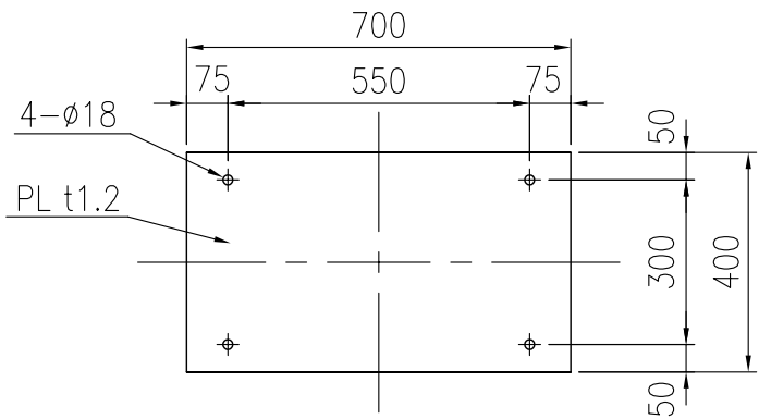
アンカーゲージ詳細図 S=1/15
