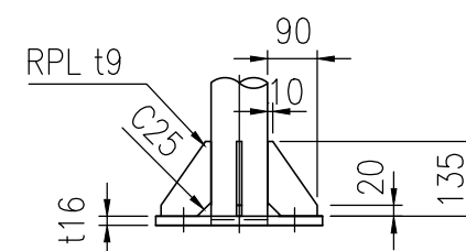
アンカーボルト詳細図 S=1/15
