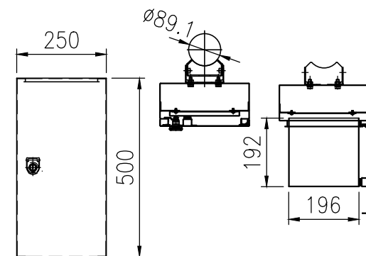
電源ボックス詳細図 S=1／15
