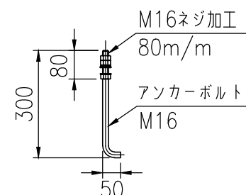
アンカーボルト詳細図 S=1／15
