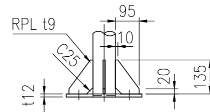
アンカーボルト詳細図 S=1／15
