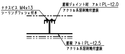
G-G断面図 (S=1:5)
