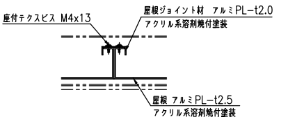
G-G断面図 (S=1:5)
