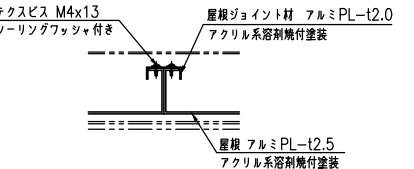
G-G断面図 (S=1:5)
