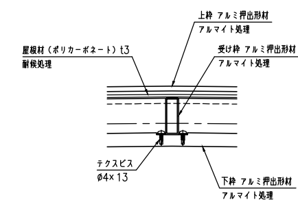
C部詳細図 (S=1:3)
