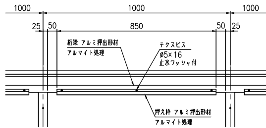
E部詳細図 (S=1:10)
