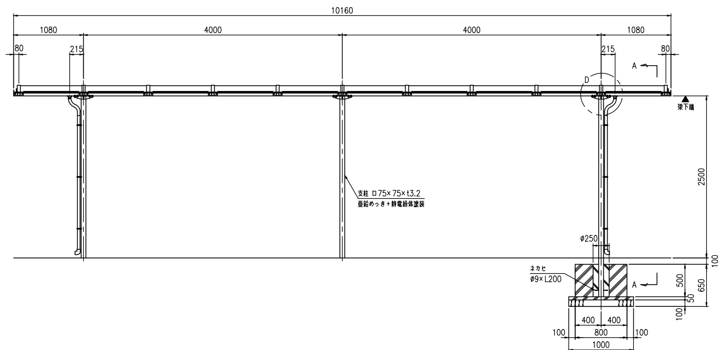
正面図 (S=1:30)
