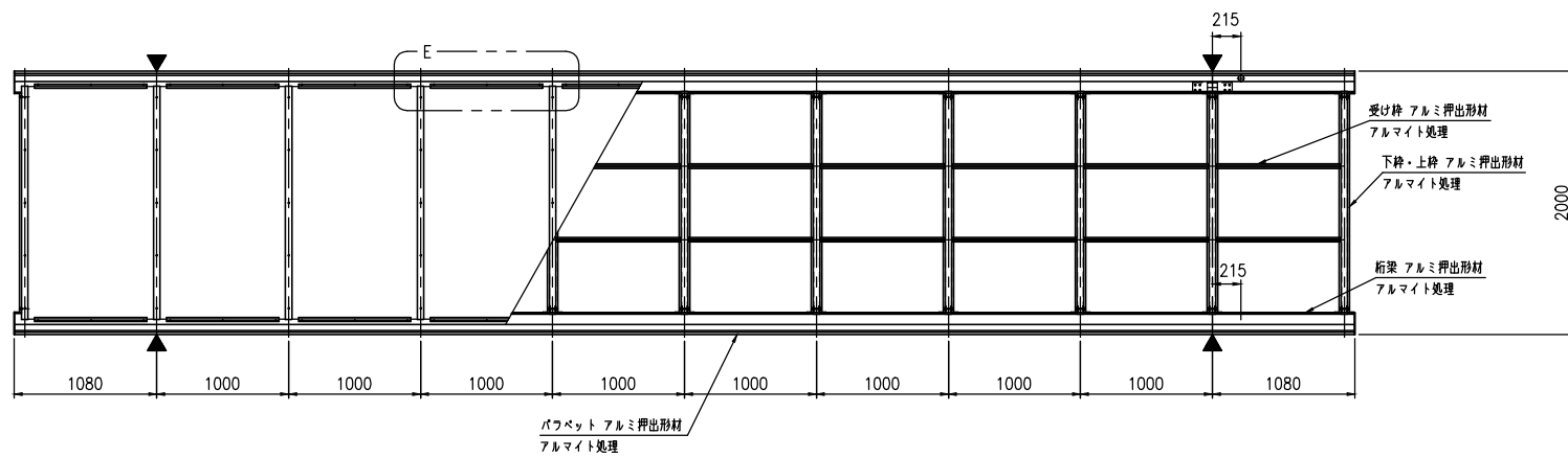
平面図 (S=1:30)
