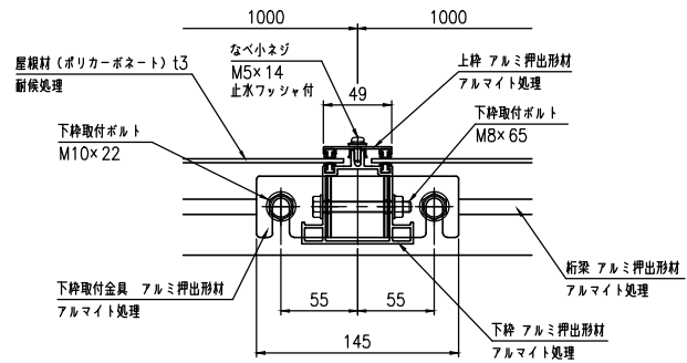
F-F断面図 (S=1:3)
