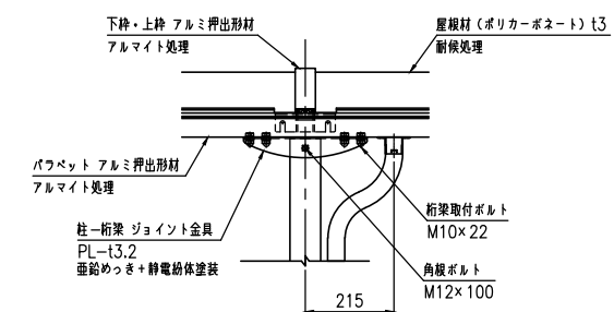
D部詳細図 (S=1:10)
