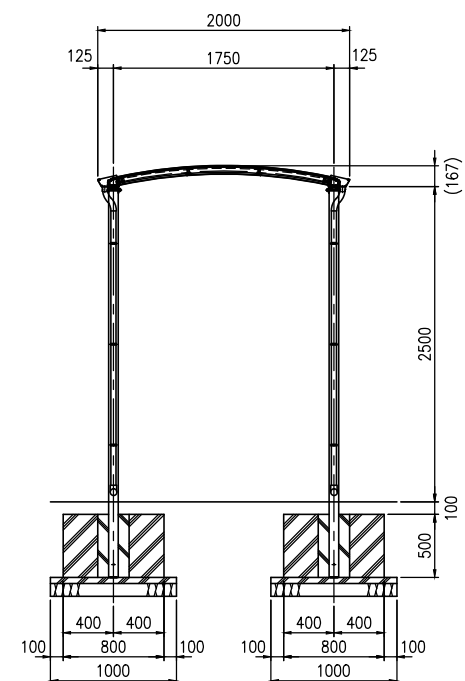
側面図 (S=1:30)
