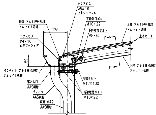
B部断面詳細図 (S=1:5)
