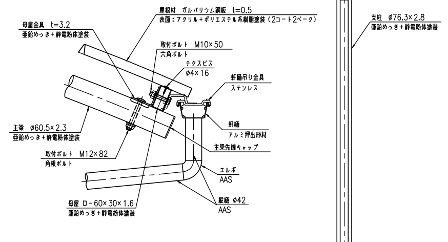
B部詳細図 (S=1:5)
