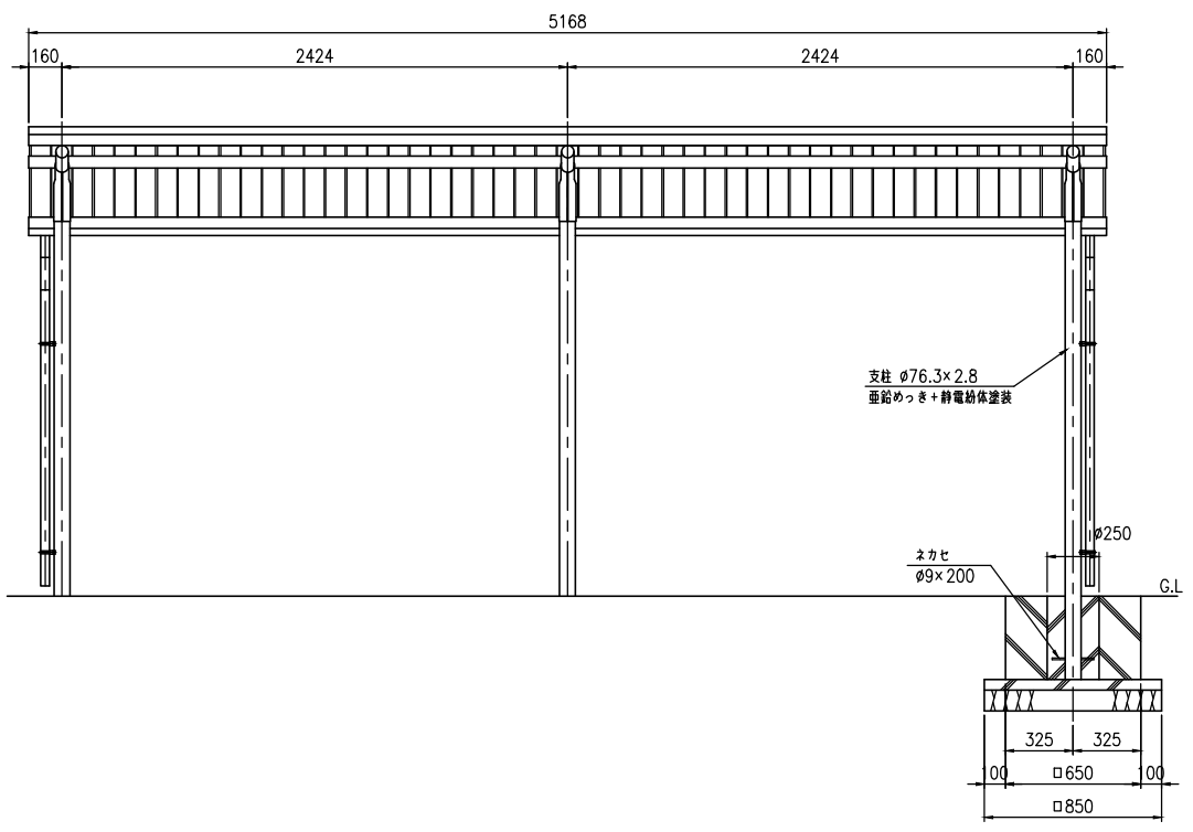
正面図 (S=1:20)
