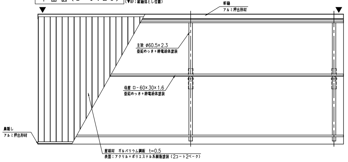
正面図 (S=1:20)
