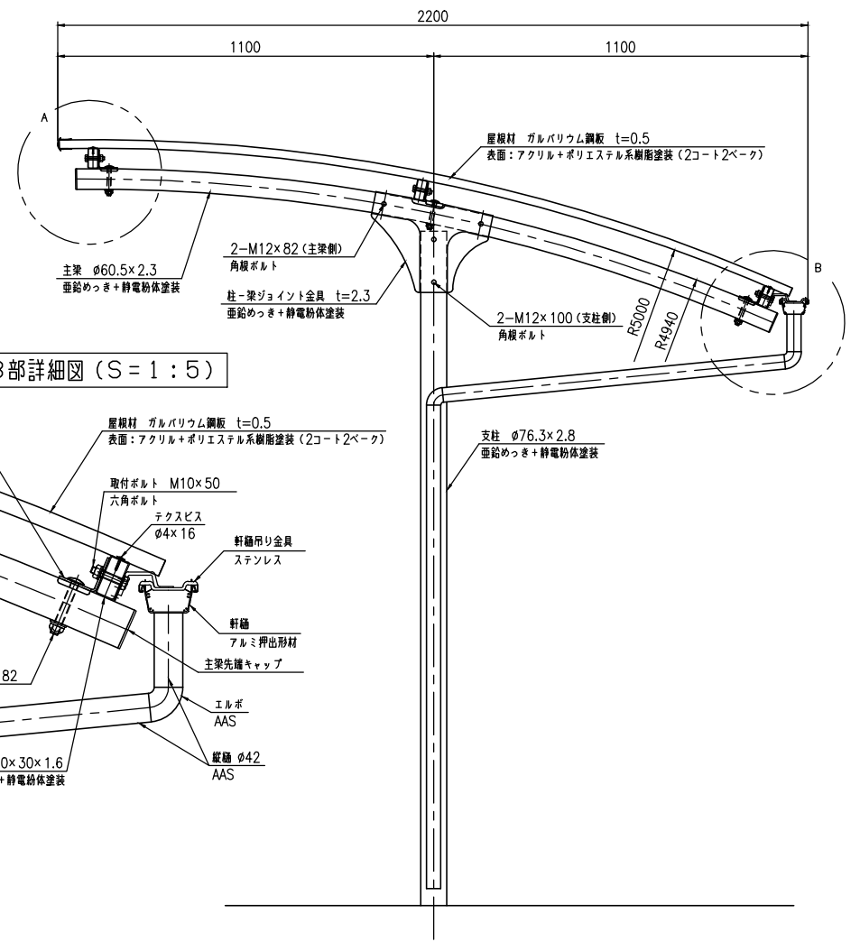
断面図 (S=1:10)
