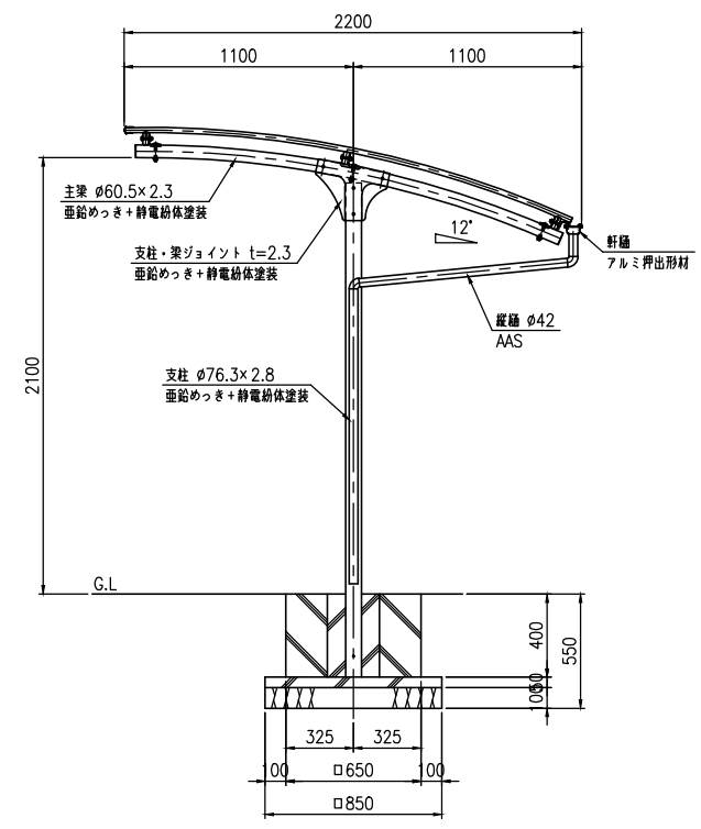
側面図 (S=1:20)
