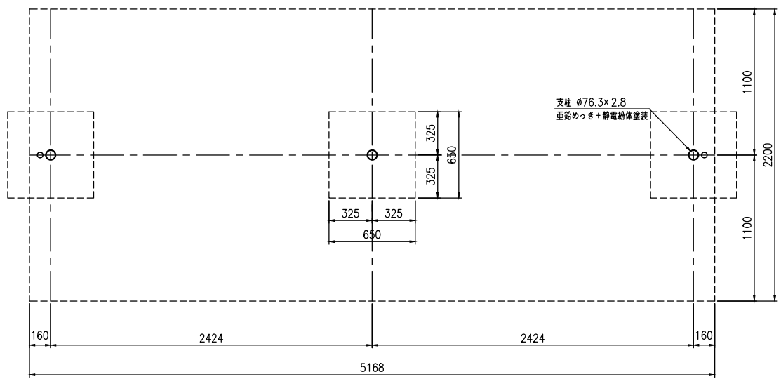
平面図 (S=1:20) (▼印: 屋根葺き位置)
