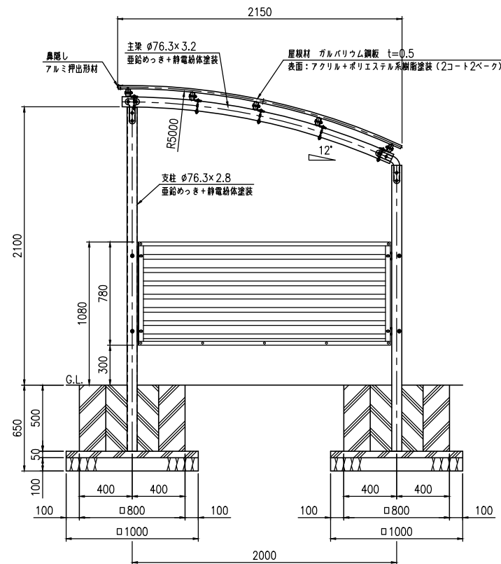
側面図 (S=1:20)
