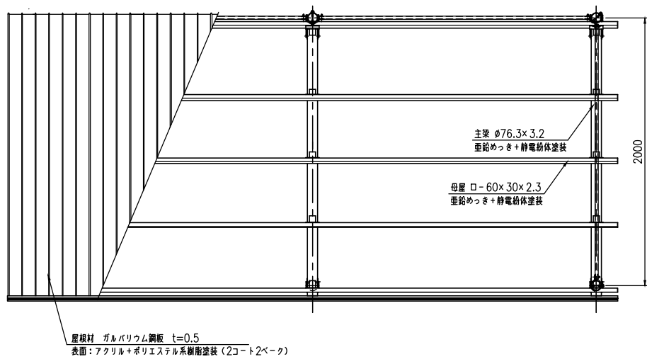
正面図 (S=1:20)
