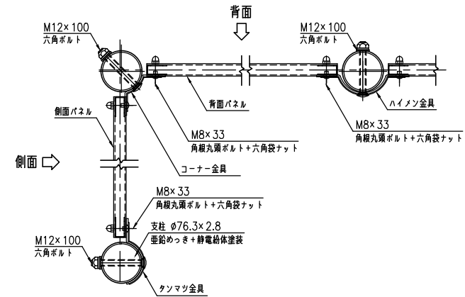
パネル取付詳細図 (S=1:5)
