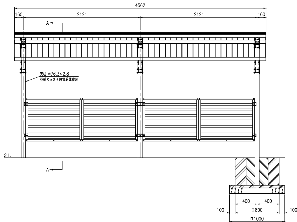
正面図 (S=1:20)
