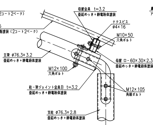
C部詳細図 (S=1:5)
