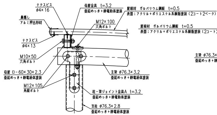
B部詳細図 (S=1:5)
