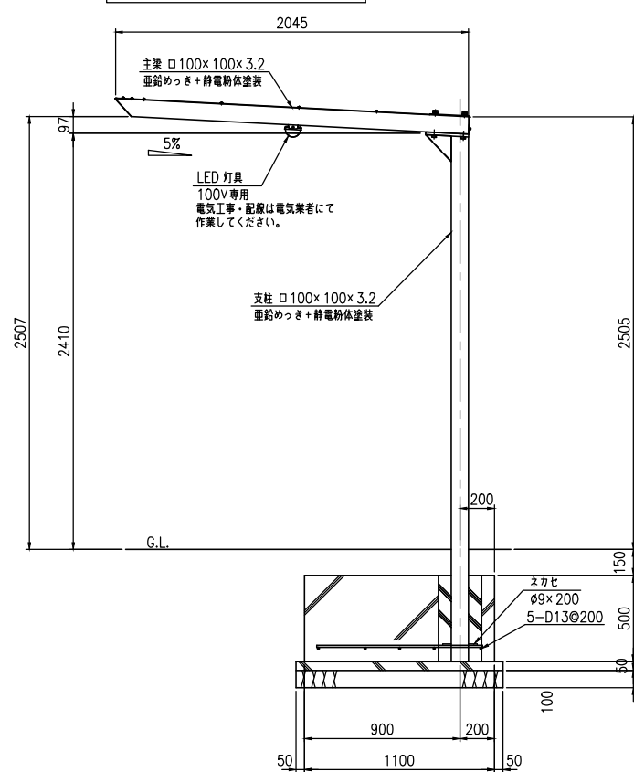
側面図 (S=1:20)
