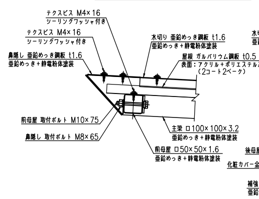
D-D断面図 (S=1:5)
