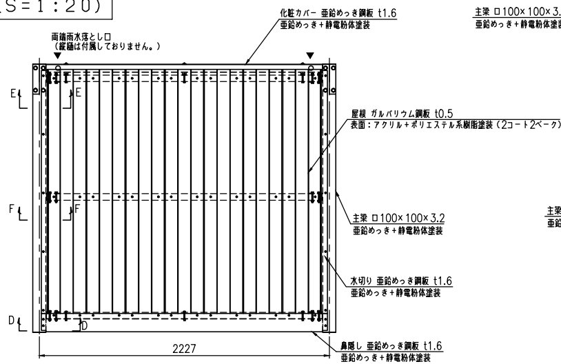
正面図 (S=1:20)
