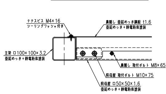
F-F断面図 (S=1:5)
