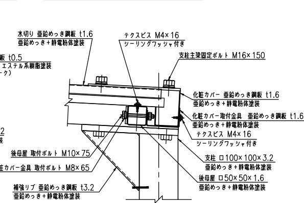
E-E断面図 (S=1:5)
