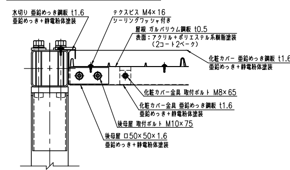
E-E断面図 (S=1:5)
