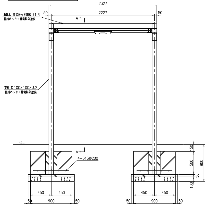
正面図 (S=1:20)
