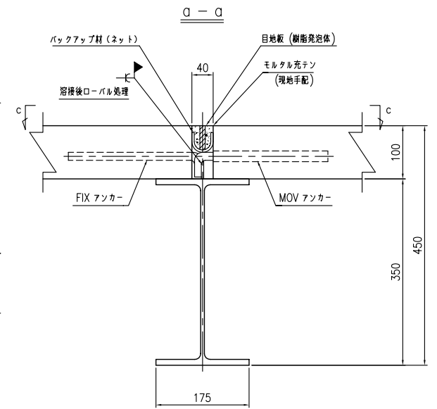
床版横目地詳細図 <S=1/5>
