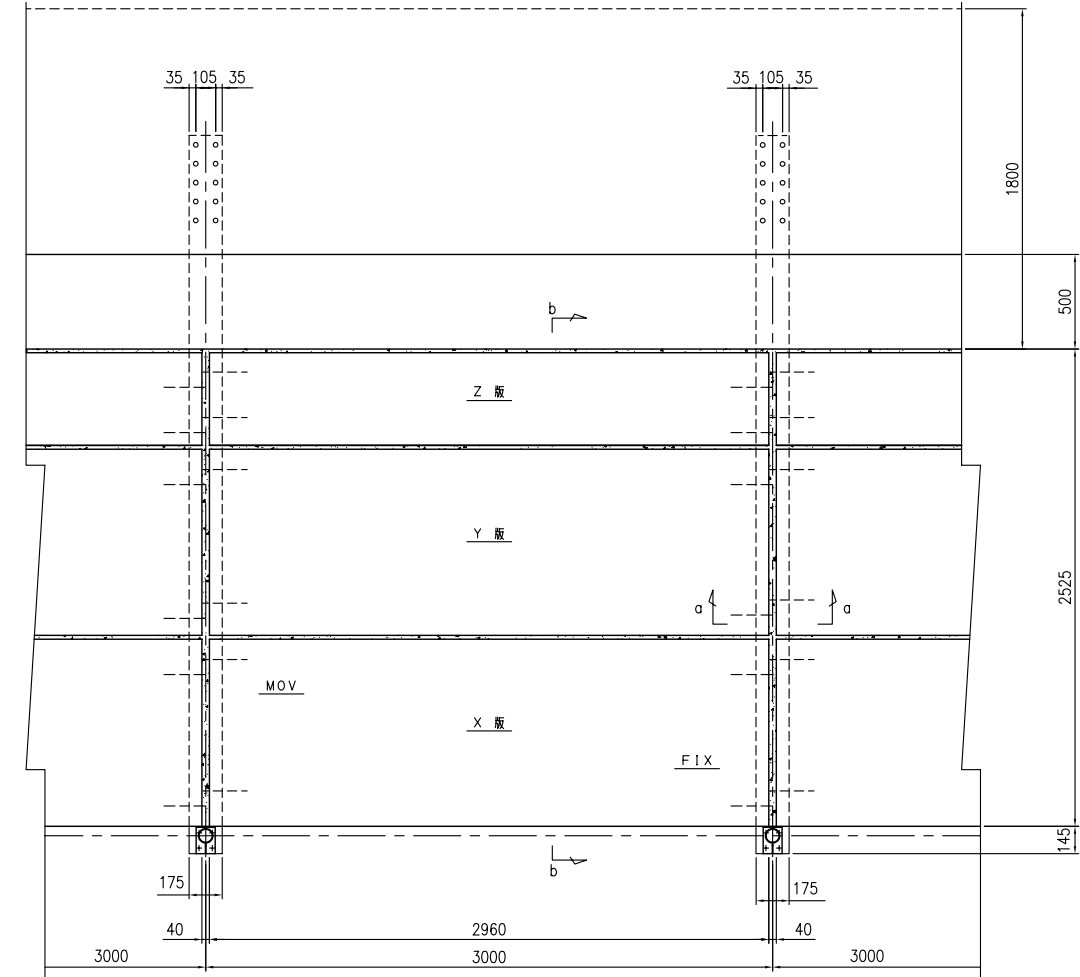
平面図 <S=1/20>
