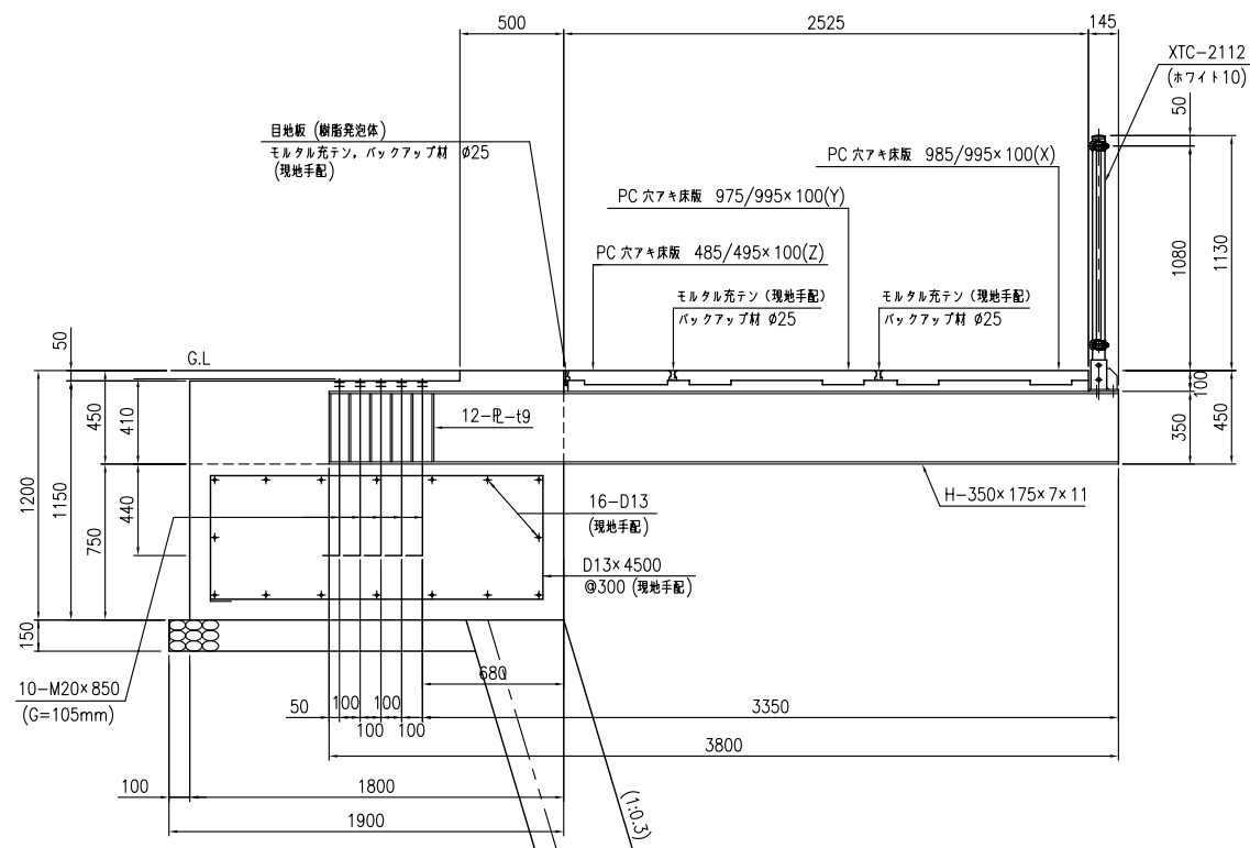
断面図 <S=1/20>
