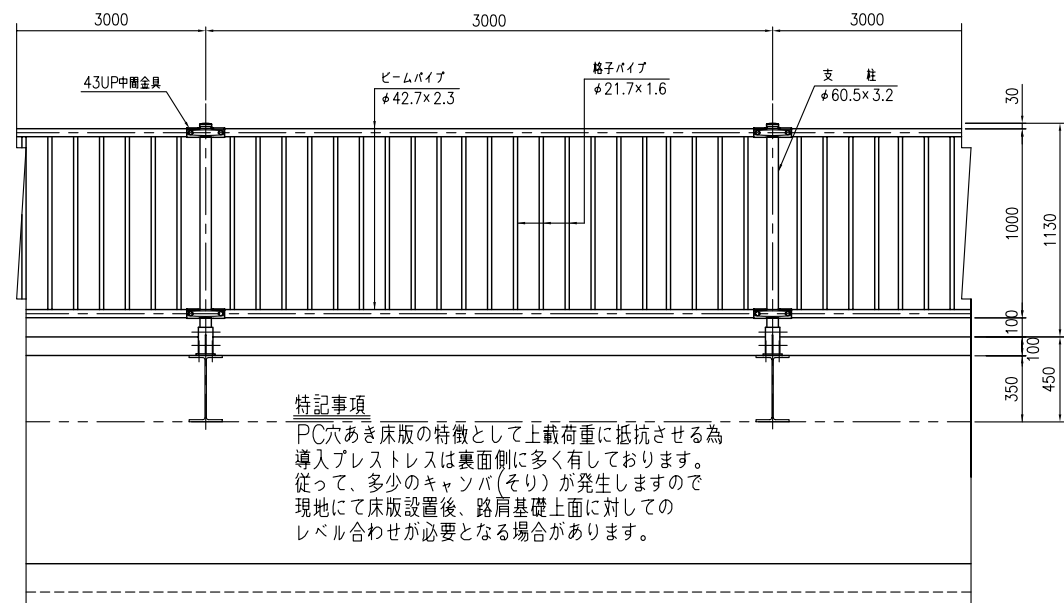
側面図 <S=1/20>
