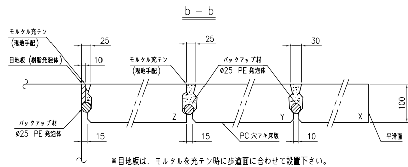
床版縦目地詳細図 <S=1/5>
