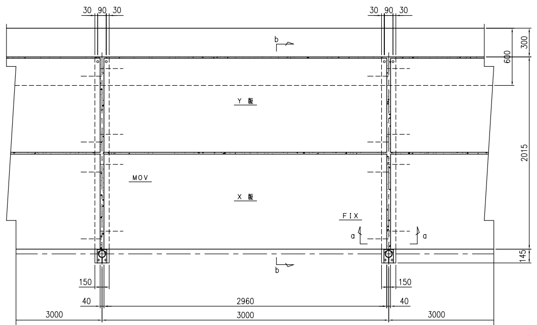
平面図 <S=1/20>
