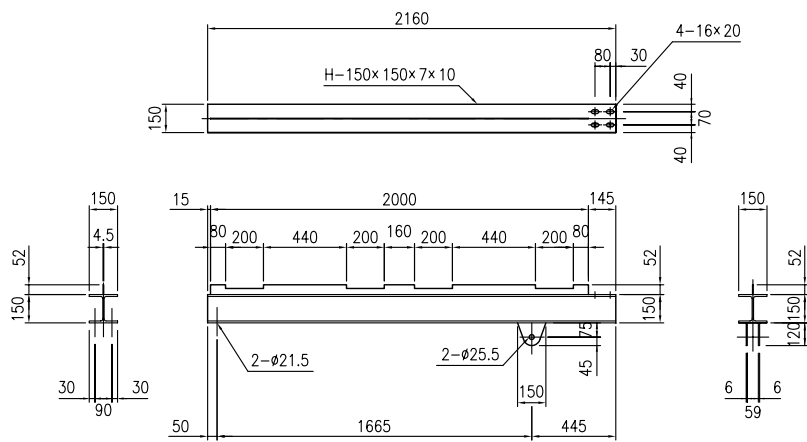
横梁詳細図 <S=1/20>
