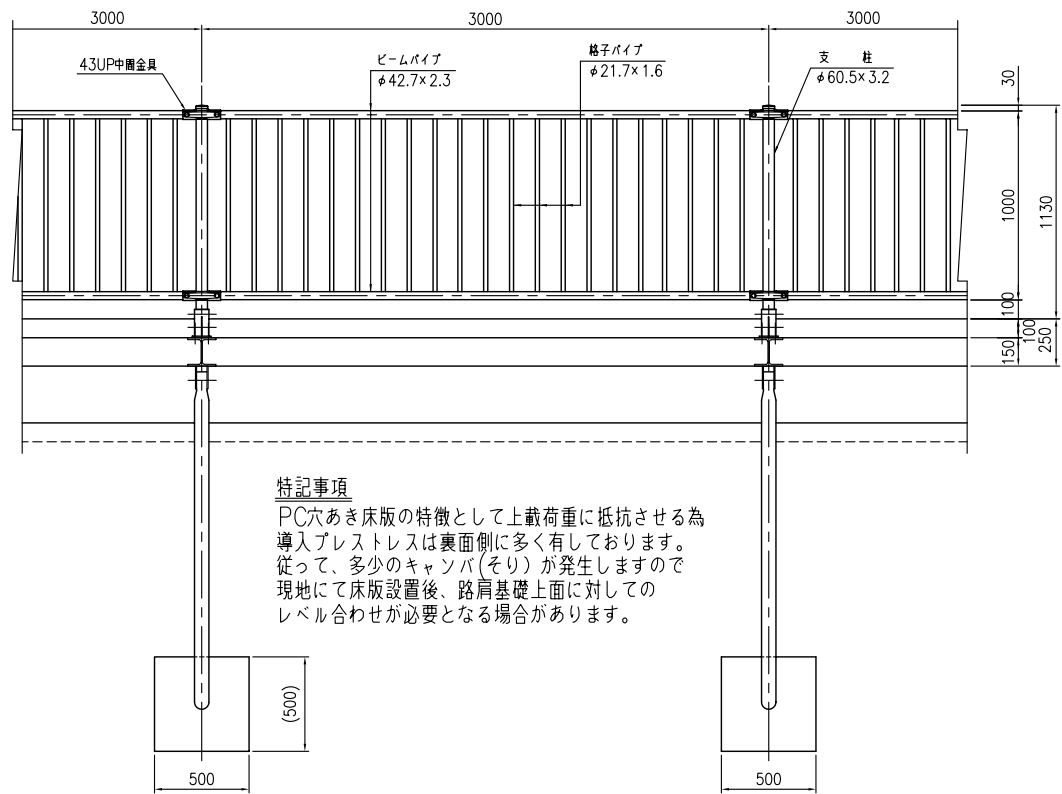
側面図 <S=1/20>
