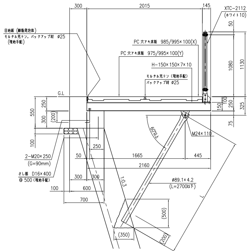
断面図 <S=1/20>
