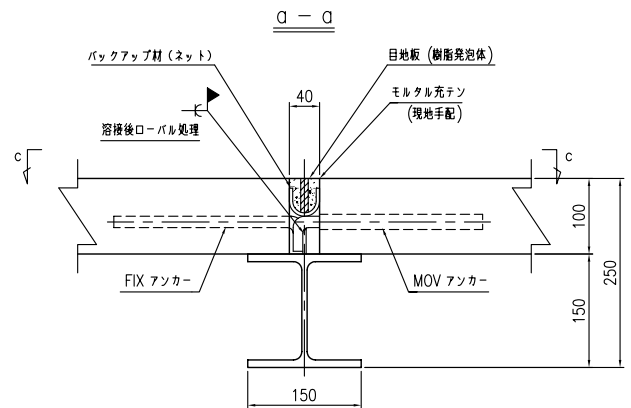
床版横目地詳細図 <S=1/5>
