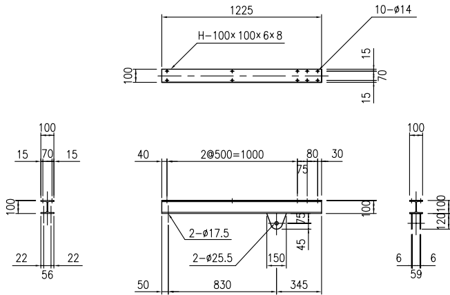
横梁詳細図 <S=1/20>
