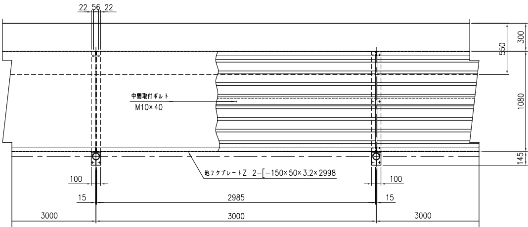
平面図 <S=1/20>
