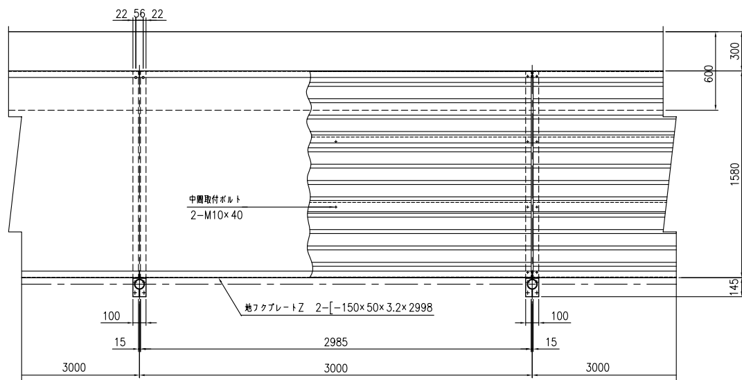
平 面 図 <S=1/20>
