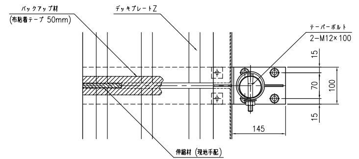
デッキプレート取付部詳細図
