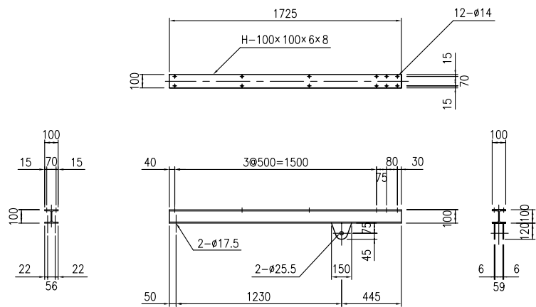
横 梁 詳 細 図 <S=1/20>
