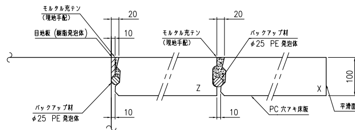
床版縦目地詳細図 <S=1/5>
