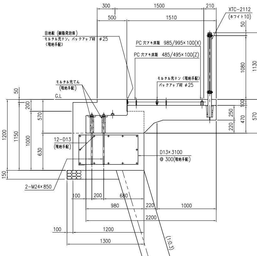
橫梁詳細図 <S=1/20>
