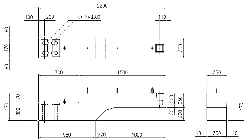
橫梁詳細図 <S=1/20>
