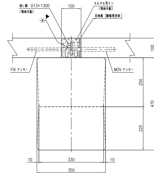
床版横目地詳細図 <S=1/5>
