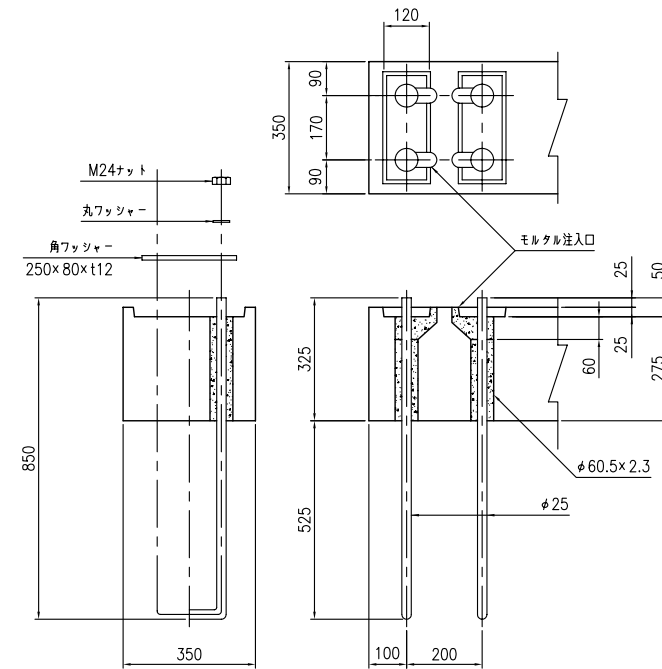
アソカーボルト埋込み部詳細図
