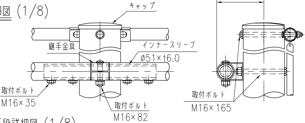
継手部最下段詳細図 (1/8)
