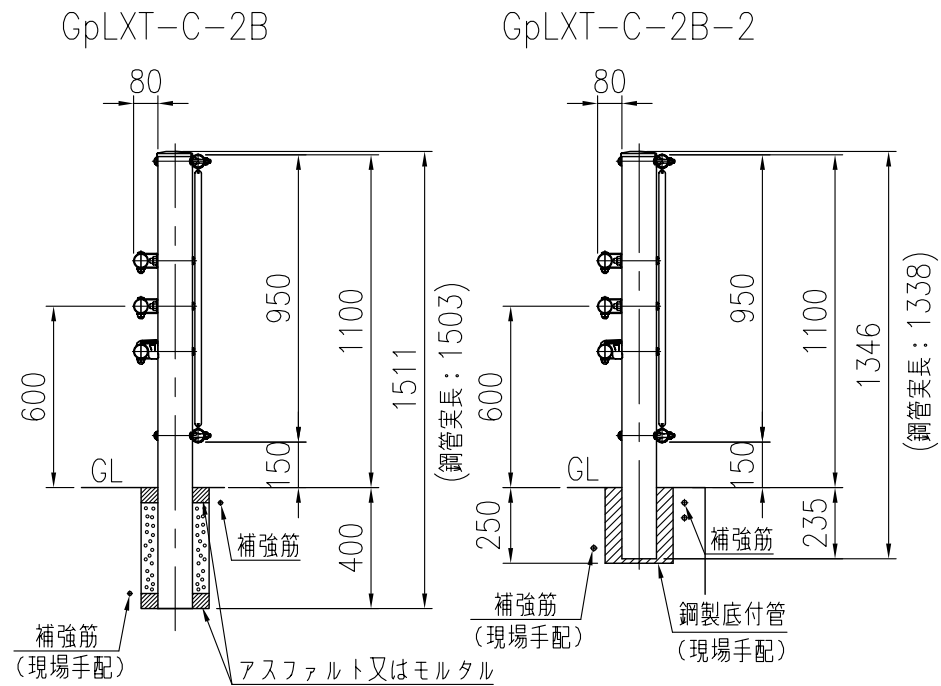
ビームパイプ詳細図 (1/10)
