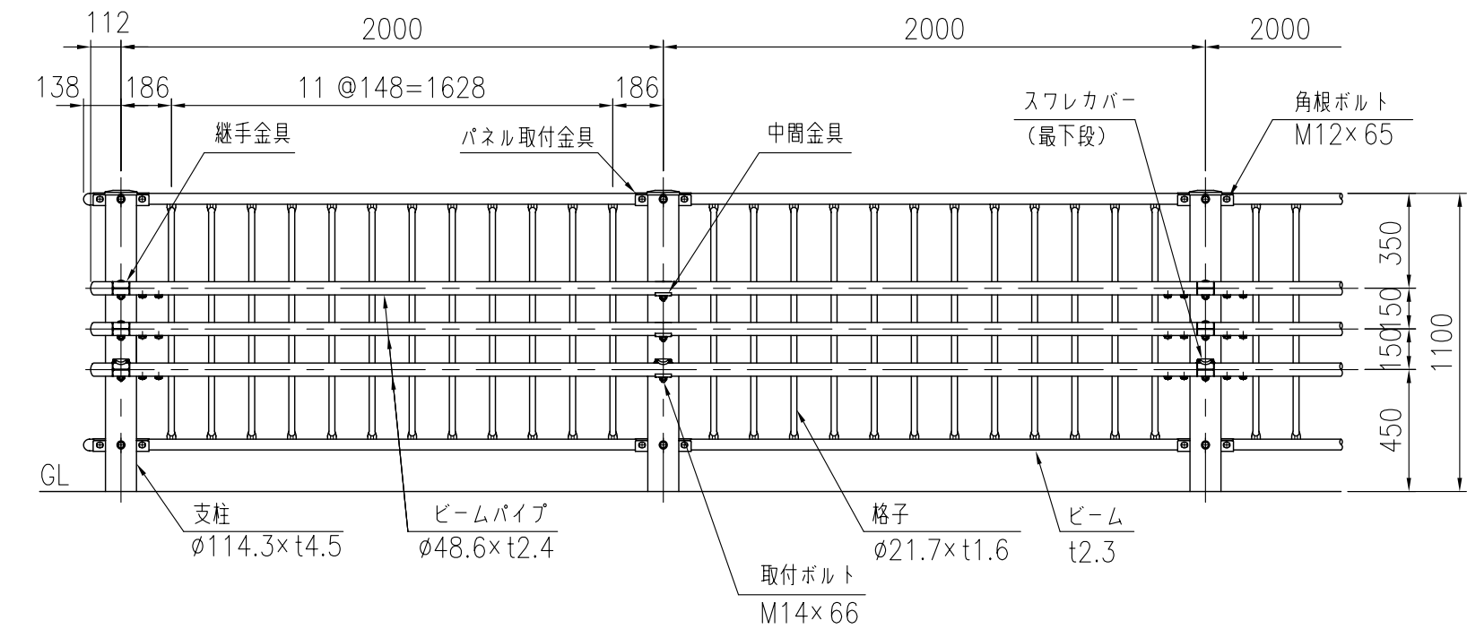
設置図 (1/25)
