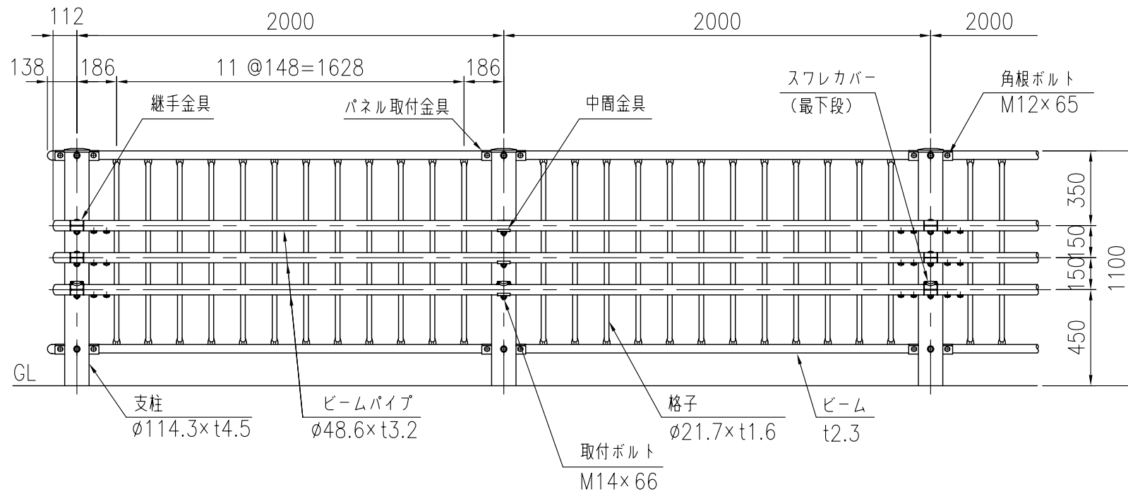
継手部詳細図 (1/6)
