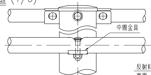
中間部最下段詳細図 (1/6)
