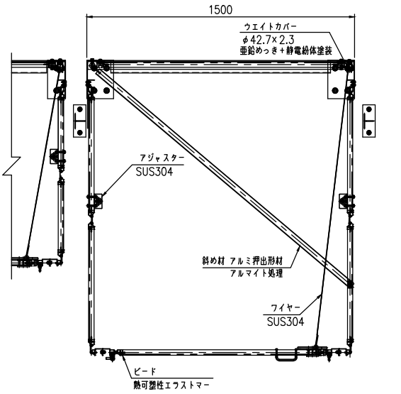
正面図 (S=1:15)
