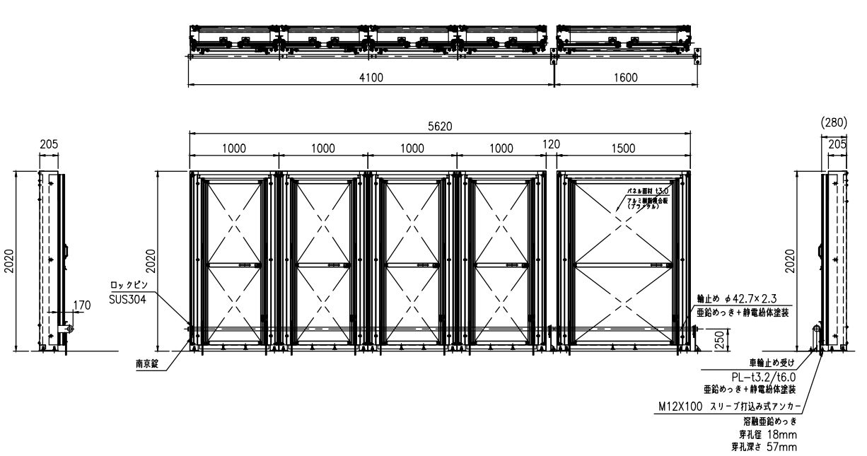
収納時 (S=1:30)
