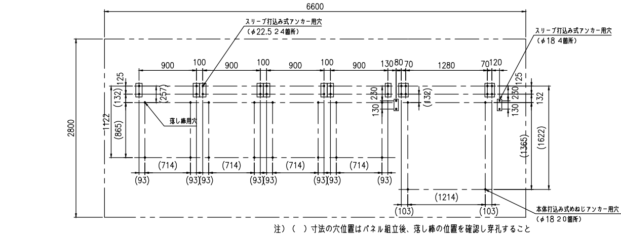
収納時 (S=1:30)
