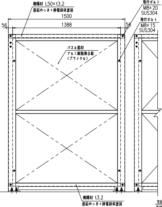
背面図 (S=1:15)
