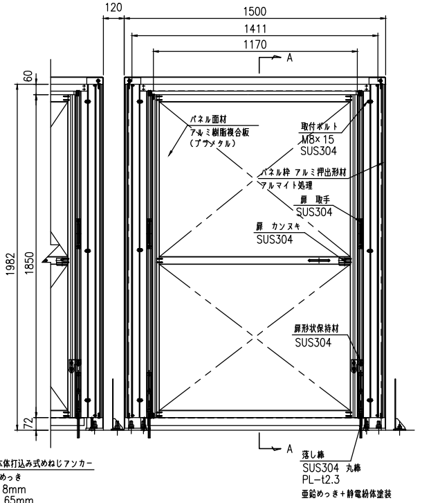
正面図 (S=1:15)
