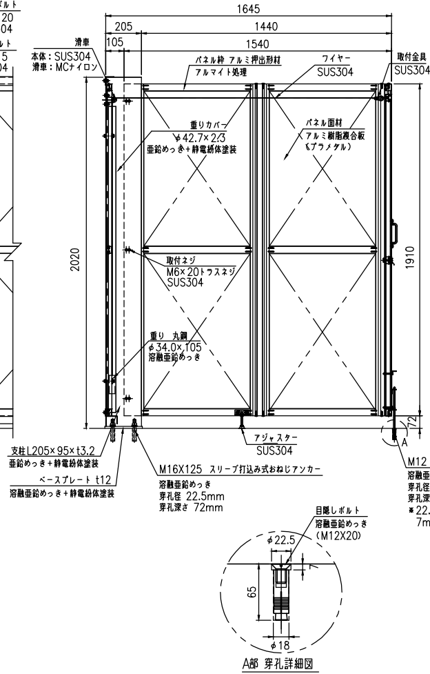
A-A断面図 (S=1:15)
