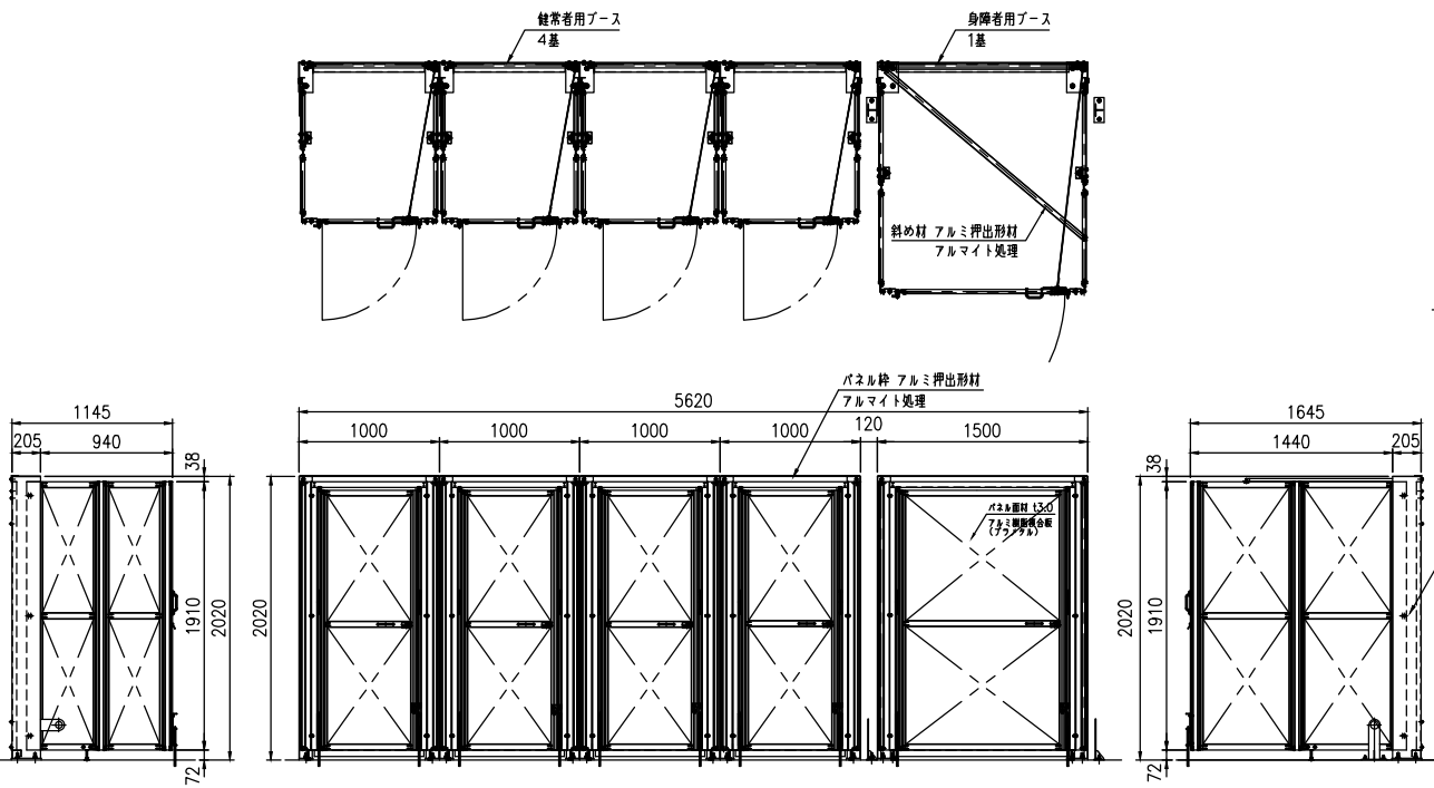
展開時 (S=1:30)
