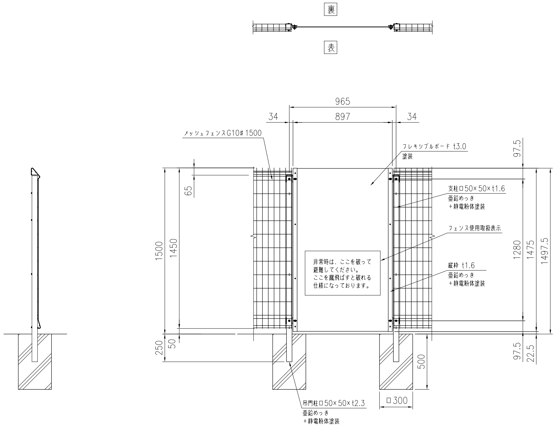
組立図 (1/20)
