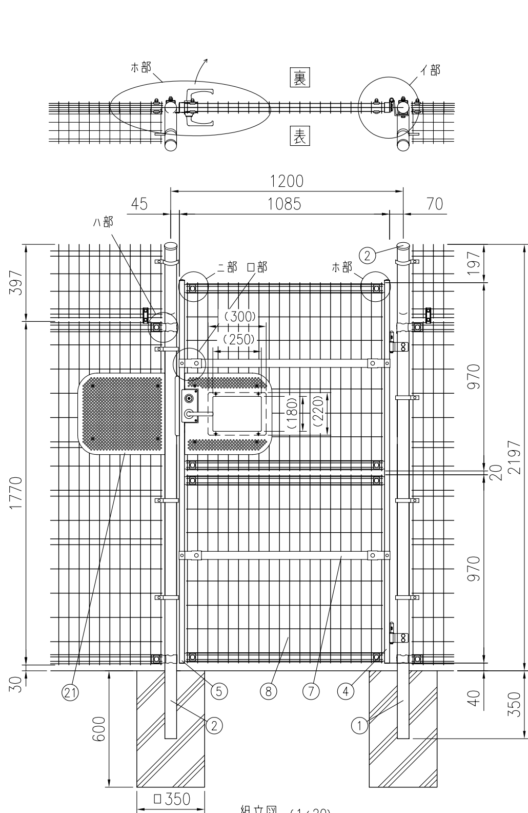
組立図 (1/20) 吊元が右、裏開きの時 注) 基礎の大きさは参考寸法です。
