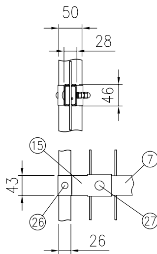
ロ部詳細図 (1/8)
