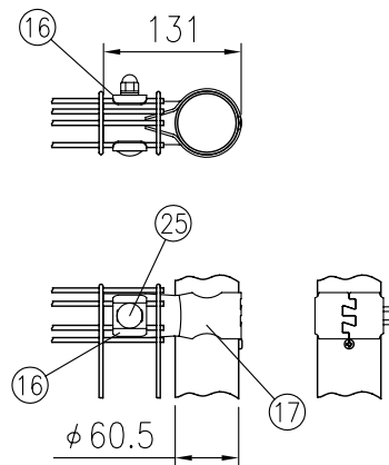
ハ部詳細図 (1/8)
