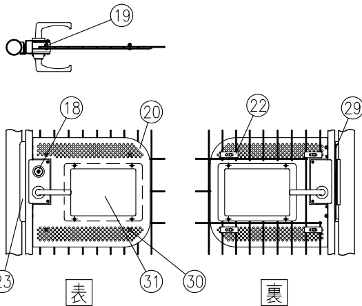
ホ部詳細図 (1/20)
