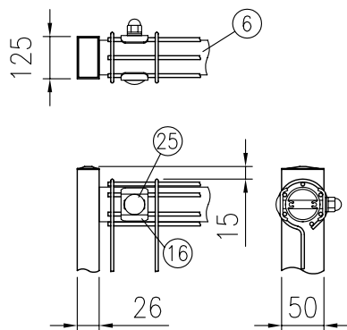
ニ部詳細図 (1/8)
