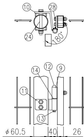
イ部詳細図 (1/8) (裏面図)
