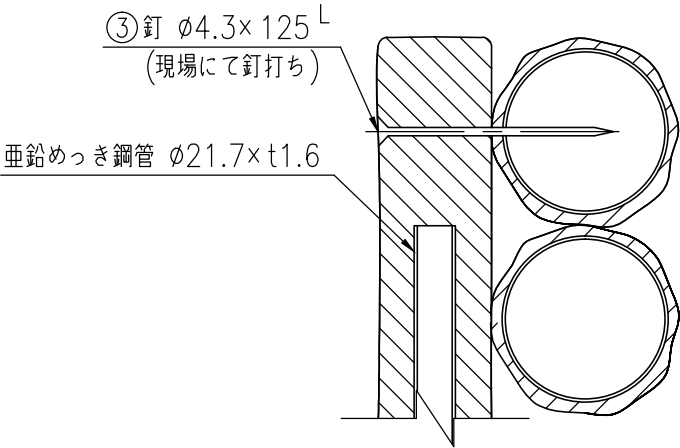
A-A'断面図 (1/4)
